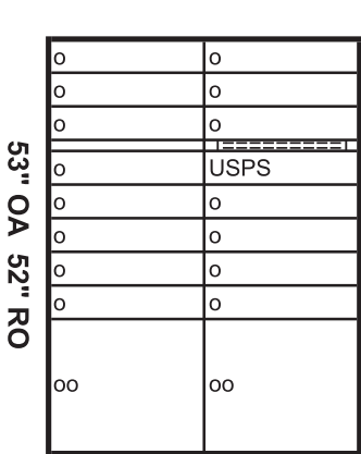
30 9/16" Model 4215-AA
