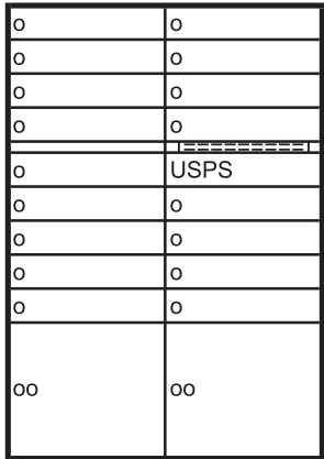
30 9/16" Model 4217-AA
